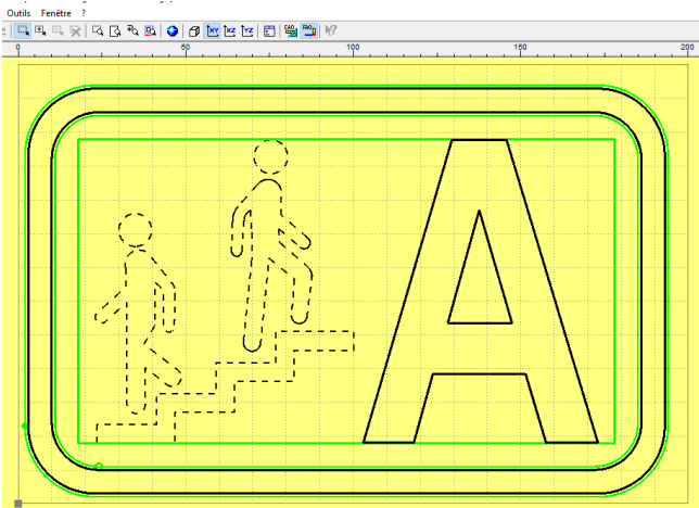
Fichier FAO pour usinage plaques escaliers
